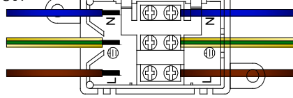
CONNECTEUR
