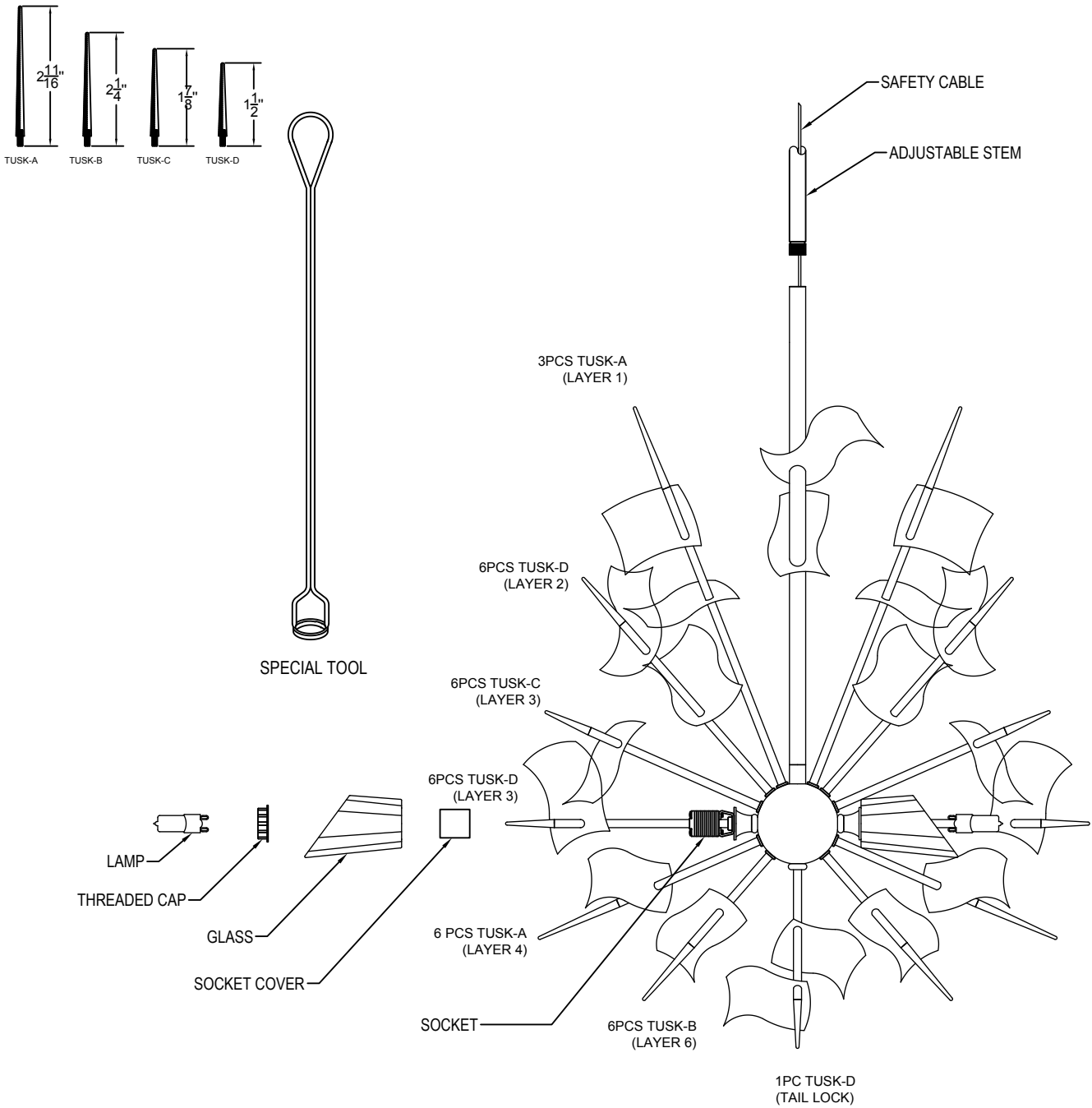
18"Ø 3-LTS. POETRY PENDANT
